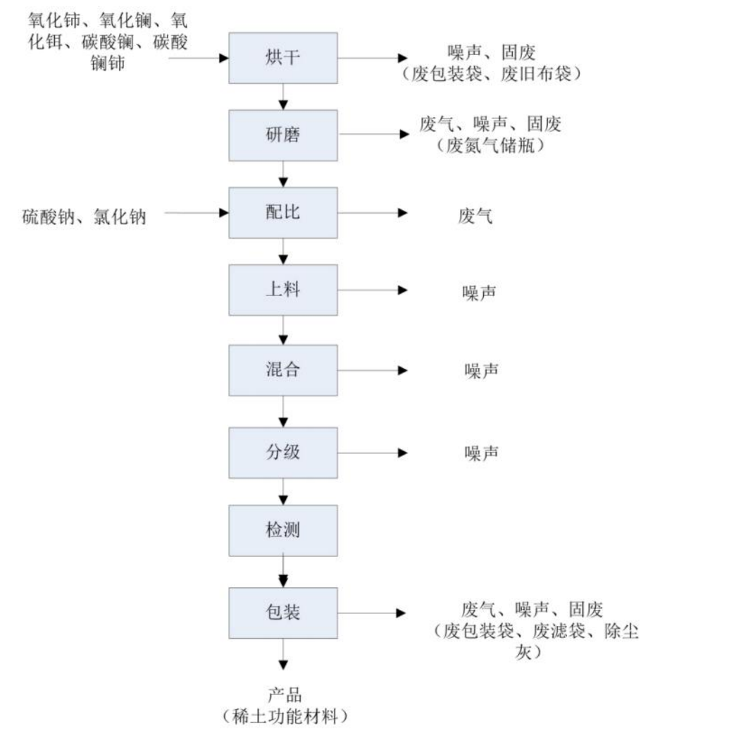
图 2-3 运营期生产工艺及产排污环节图
