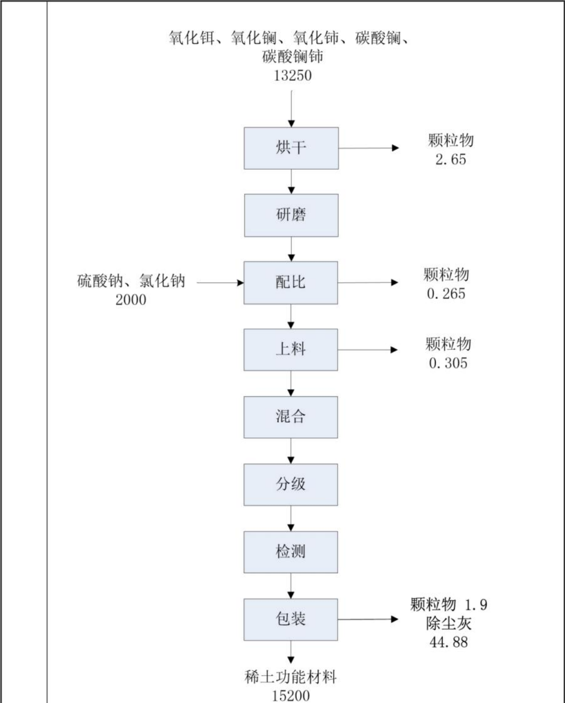
图 2-1 本项目物料平衡图 单位：t/a
