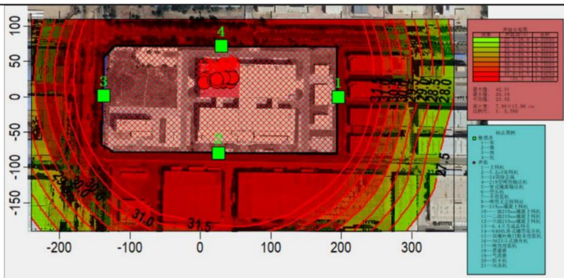
图 4-3 噪声预测结果图
