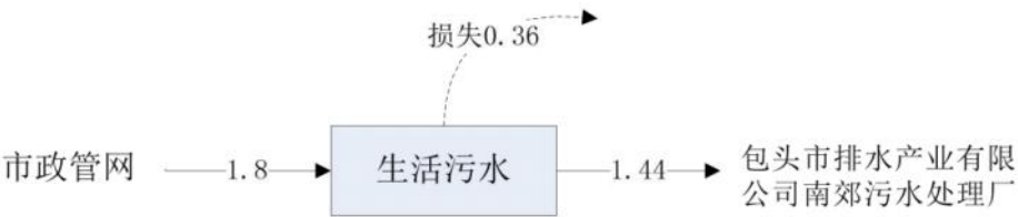
图 2-2 本项目水平衡图（单位 m³/d）
