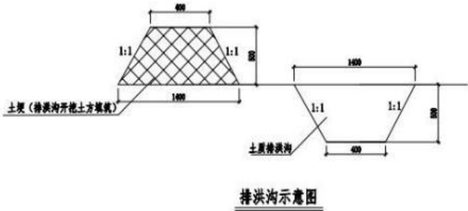
图 2-2 截洪沟示意图
